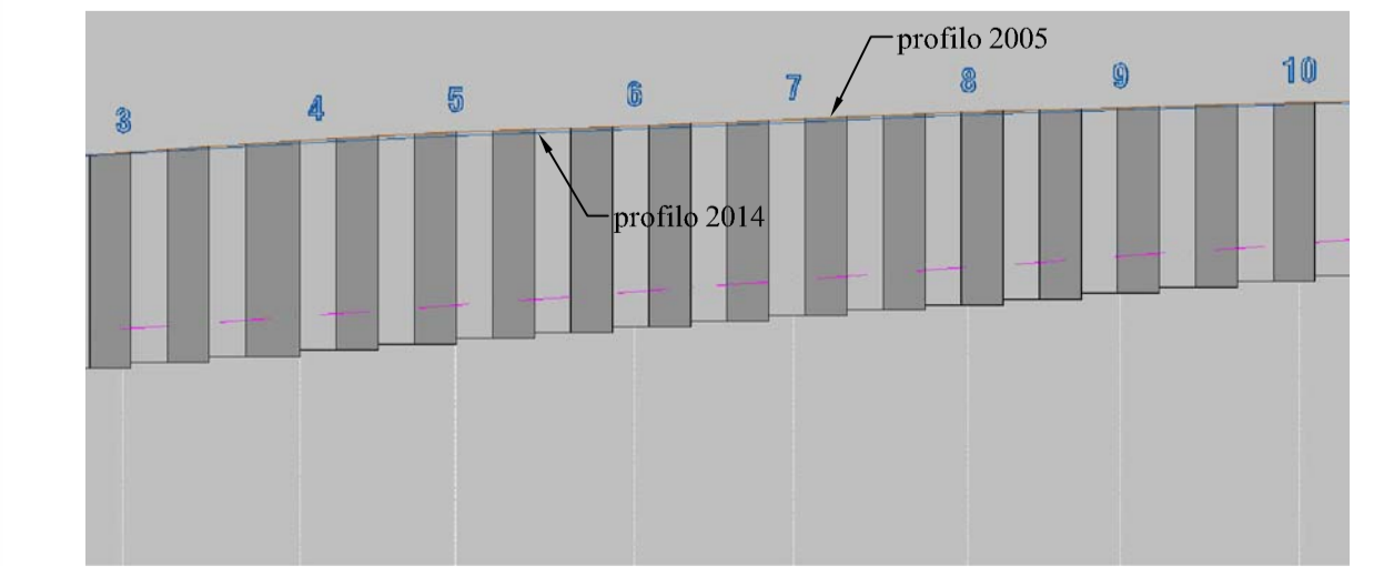
Tratto del profilo longitudinale del diaframma dove si concentrano le maggiori differenze tra i rilievi 2005 e 2014
